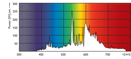
MASTERCouleur CDM-R Elite 70W /930 PAR30L
