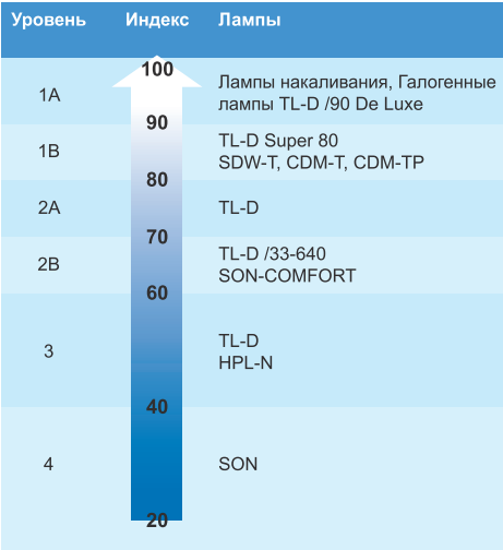
ИНДЕКС ЦВЕТОПЕРЕДАЧИ
