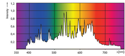
MASTERCouleur CDM-TMW Elite 315W/942
