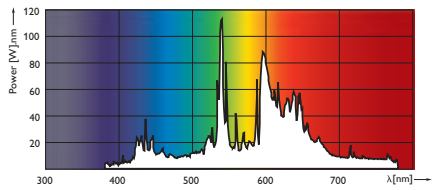
MASTERCouleur CDM-R Elite 35W /930 PAR30L
