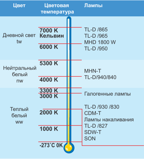
ЦВЕТОВАЯ ТЕМПЕРАТУРА
