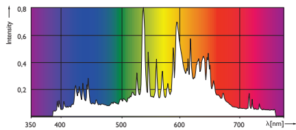
MASTERCouleur CDM-TMW Elite 210W/930
