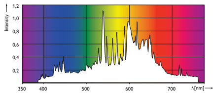
MASTERCouleur CDM-TMW Elite 315W/930
