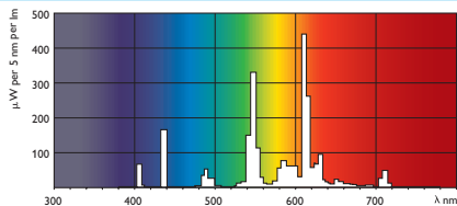
Цвет излучения 827
