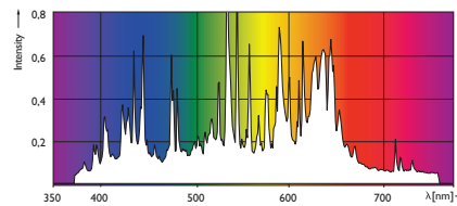
MASTERCouleur CDM-TMW Elite 210W/942
