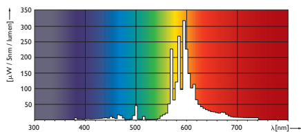
SON | 50W & 70W
