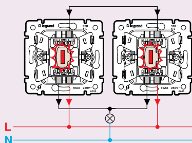
Управление из 2 мест: переключатель на 2 направления с подсветкой 7743 25 (7744 25)
