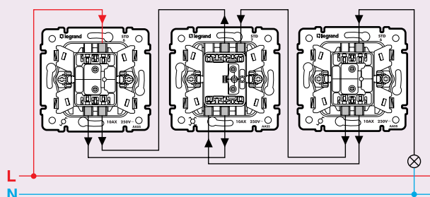
Управление из 3 мест: 2 переключателя на 2 направления и промежуточный переключатель 7743 06 + 7743 07 + 7743 06 (или 7744 06 + 7744 07 + 7744 06)
