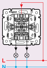
Двойной выключатель 7743 05 (7744 05)
