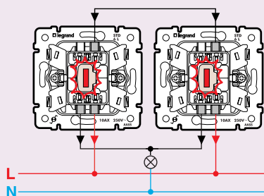
Управление из двух мест: переключатель на 2 направления с подсветкой 7743 26 (7744 26)
