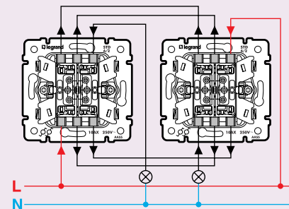
Управление из 2 мест 2-мя группами светильников: переключатель на 2 направления 7743 08 (7744 08)
