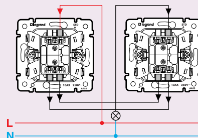
Управление из 2 мест: переключатель на 2 направления 7743 06 (7744 06)
