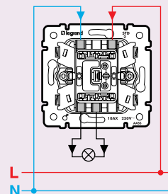
Двухполюсный выключатель 7743 02 (7744 02)
