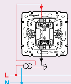
Выключатель кнопочный 7743 11 (7744 11)
