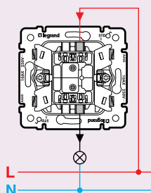
Выключатель 7743 01 (7744 01)
