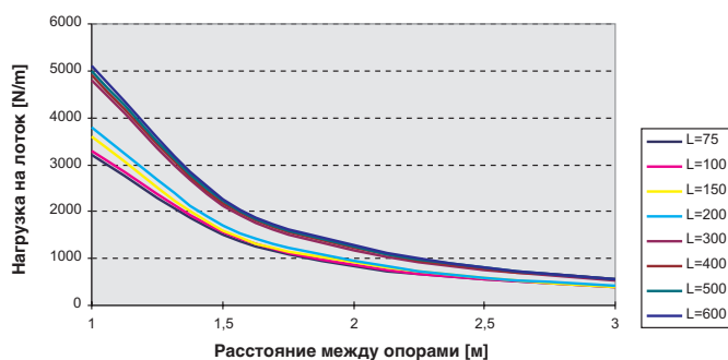
КАБЕЛЬНЫЕ ЛОТКИ P31 H75
