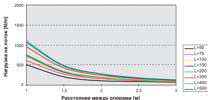
КАБЕЛЬНЫЕ ЛОТКИ P31 H25
