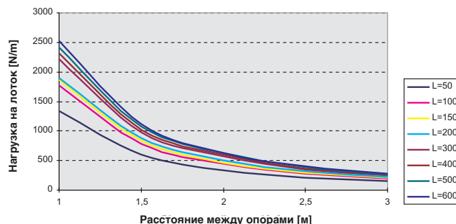
КАБЕЛЬНЫЕ ЛОТКИ P31 H50
